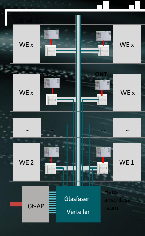
Inhausverkabelung in einem Mehrfamilienhaus
